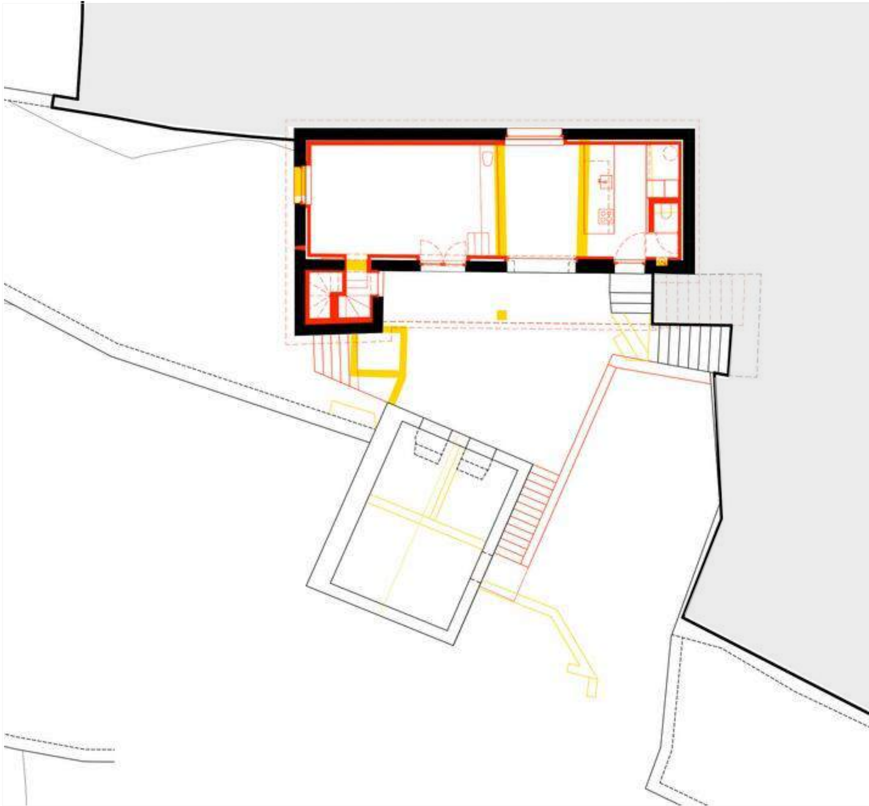
PLANTA DO RÉS-DO-CHÃO - CC
