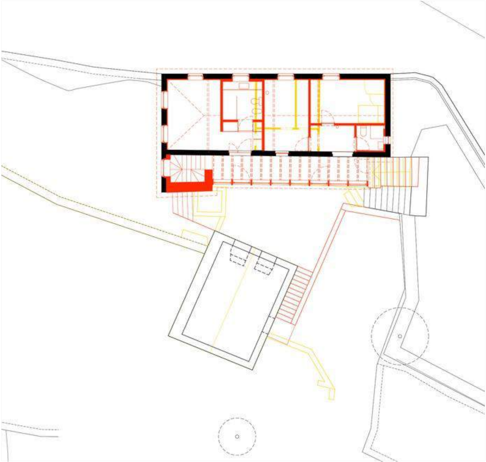
PLANTA DO 1º ANDAR - CC
